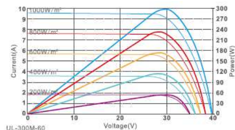
I-V charakterystyka
